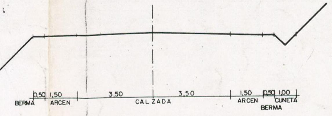
SECCION VIAL TIPO
